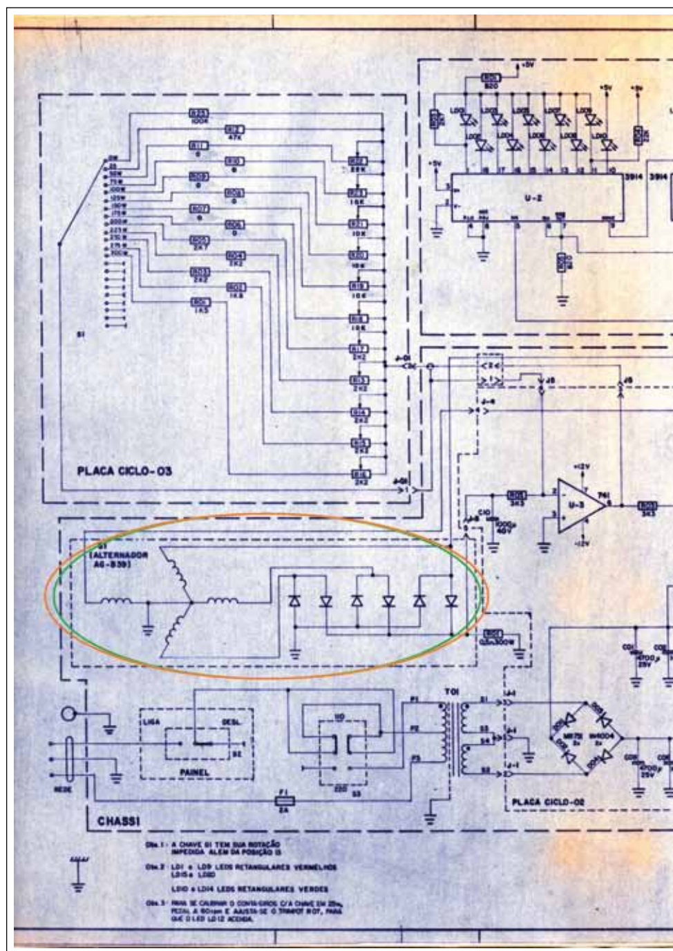
Esquema elétrico do sistema de frenagem eletromagnética, empregado nos primeiros cicloergômetros da FUNBEC, no início da década de 70. Foto gentilmente cedida por Eric Delisle.
